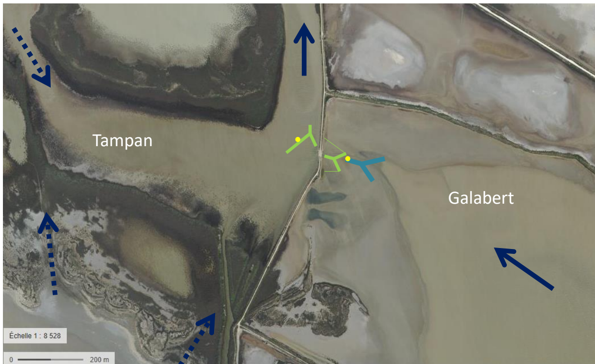
Figure A2-52 : Plan du dispositif de pêche à l'ouvrage de connexion entre les étangs du Galabert 2 et du Tampan pour le suivi d'octobre 2016 à Juin 2017. Les flèches bleues marines en trait continu indiquent le cheminement pour remonter le système en direction de l'étang du Vaccarès. Les flèches en trait discontinu illustrent les connexions possibles avec la mer en cas d'avis de grand frais de secteur Sud. Les points jaunes symbolisent le positionnement des sondes d'enregistrement des niveaux d'eau. Le filet DCE est schématisé en bleu clair et les filets à civelles en vert. Photo satellite de Géoportail © IGN 2017
