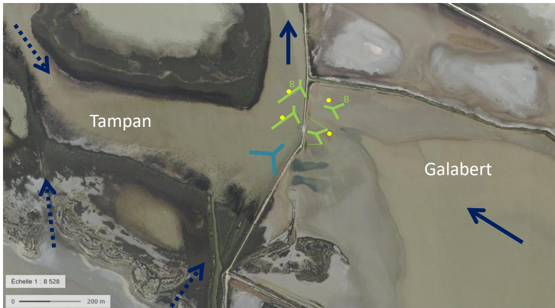
Figure A2-58 : Plan du dispositif de pêche à l'ouvrage de connexion entre les étangs du Galabert 2 et du Tampan pour le suivi à partir d'octobre 2019. Les flèches bleues marines en trait continu indiquent le cheminement pour remonter le système en direction de l'étang du Vaccarès. Les flèches en trait discontinu illustrent les connexions possibles avec la mer en cas d'avis de grand frais de secteur Sud. Les points jaunes symbolisent le positionnement des sondes d'enregistrement des niveaux d'eau. Le filet DCE est schématisé en bleu clair et les filets à civelles en vert. Photo satellite de Géoportail © IGN 2017. Le nouvel ouvrage et son chenal ne sont pas encore visibles.
