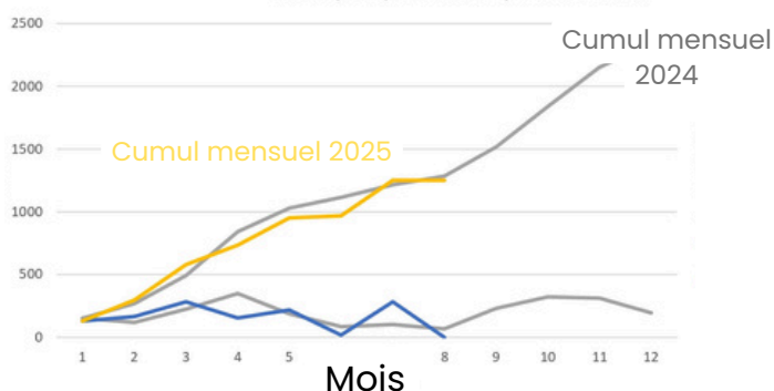
Cumul précipitations 11 pour 5 stations
